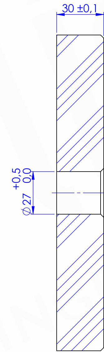
COUPE A-A
