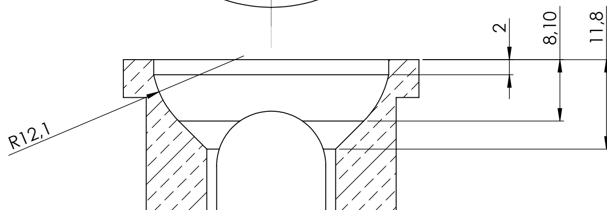
COUPE E-E ECHELLE 2 : 1
