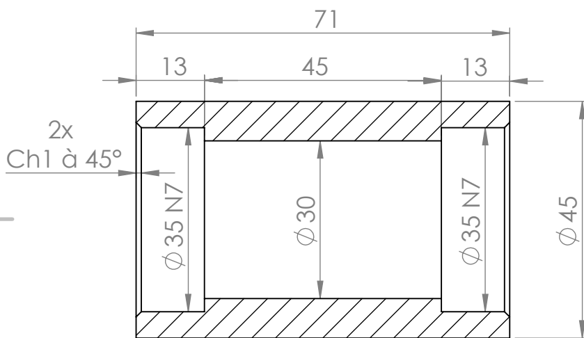
COUPE A-A
