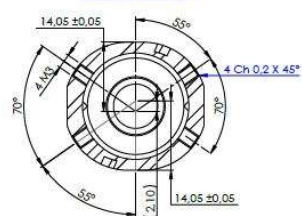
COUPE B-B
