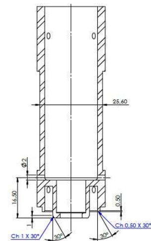
COUPE E-E
