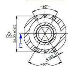
COUPE D-D
