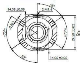
COUPE C-C
