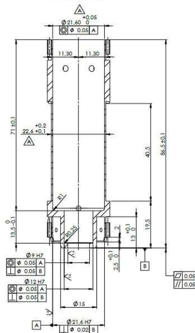
COUPE A-A
