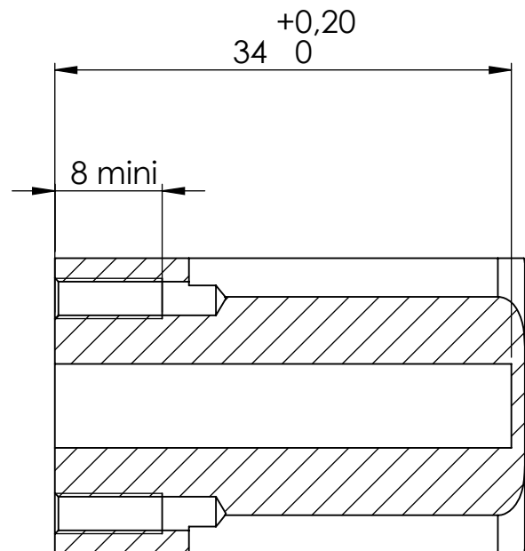
COUPE B-B
