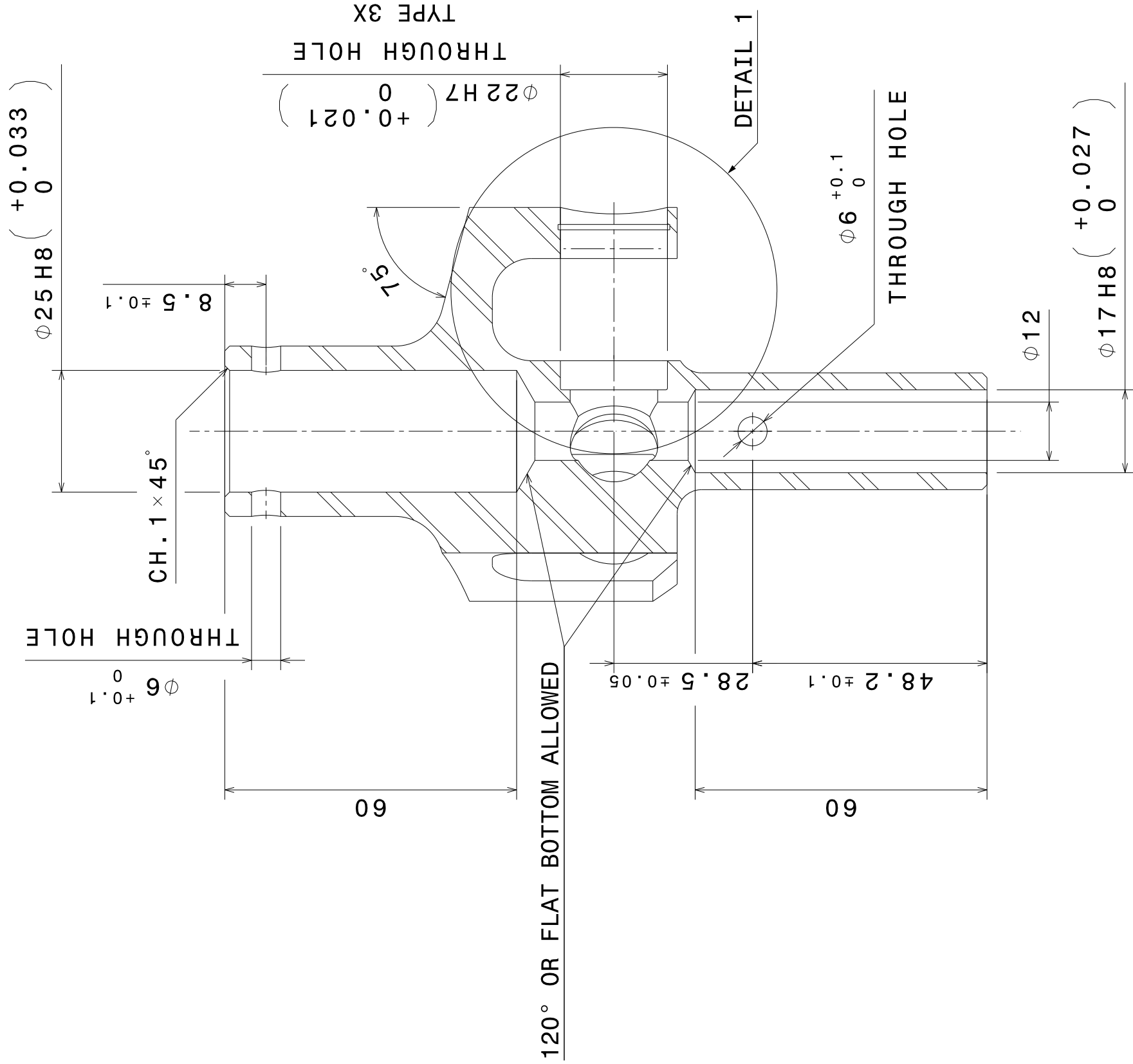
Section view A-A Scale: 1:1
