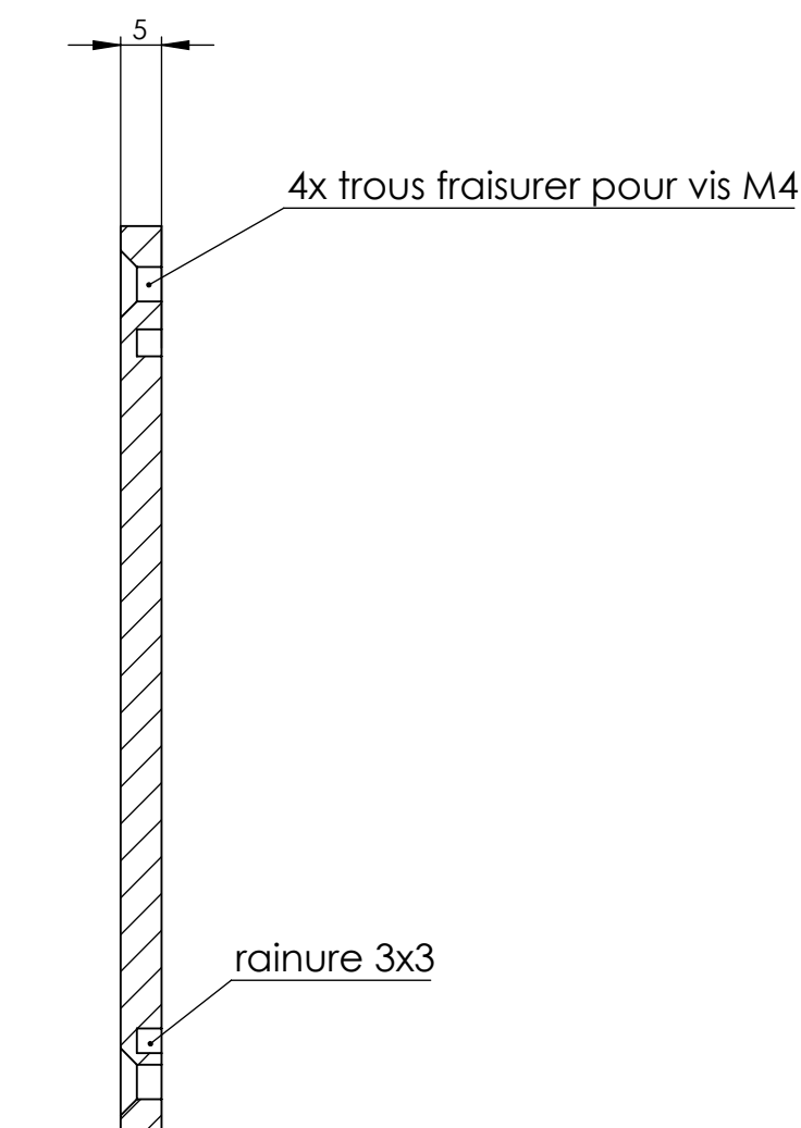
COUPE O-O ECHELLE 1 : 1
