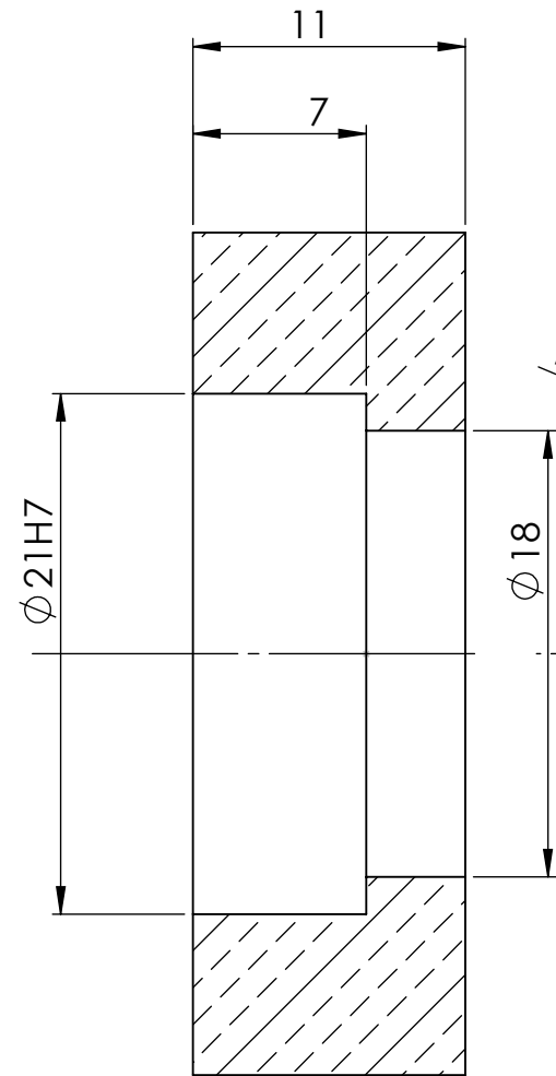
COUPE A-A ECHELLE 3 : 1
