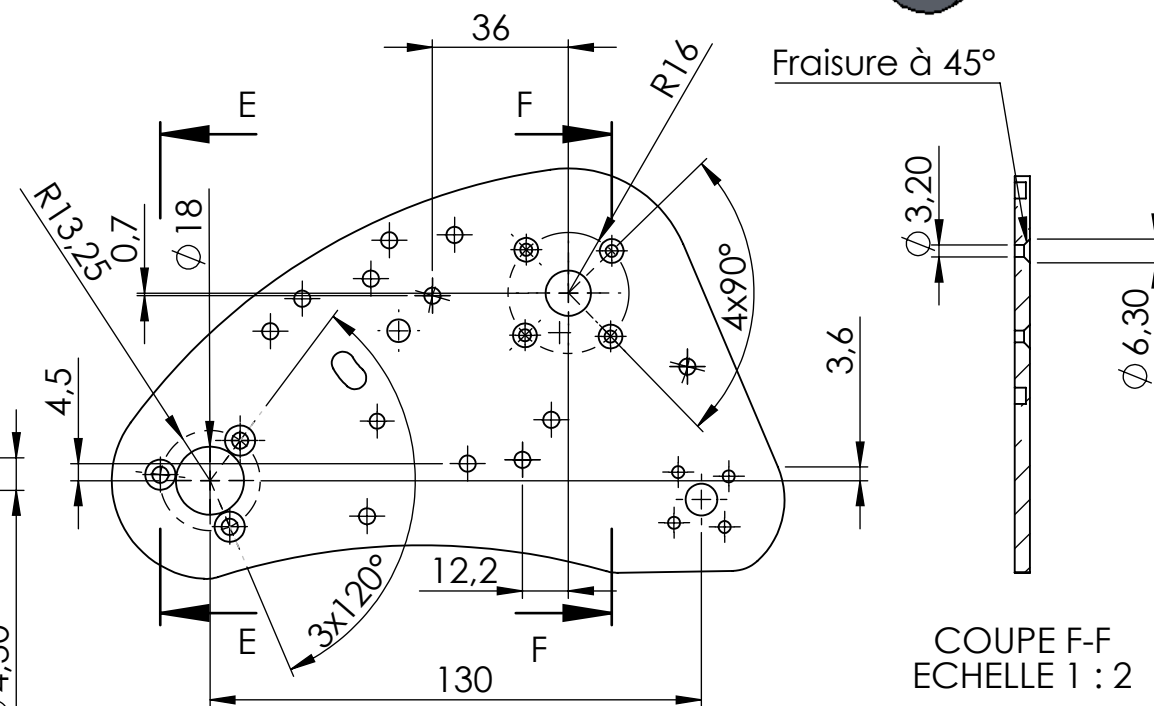
COTES NON DEFINIES ET FORME SUIVANT CAO
