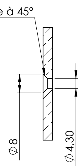
COUPE E-E
