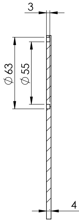
COUPE C-C
