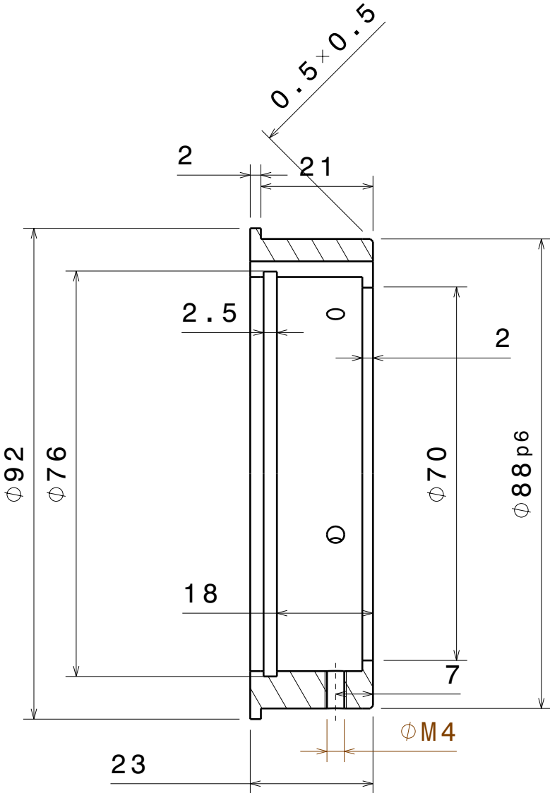
Coupe A-A Echelle : 1:1
