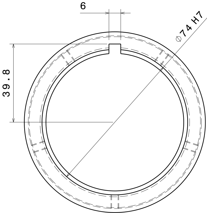
Vue de dos Echelle : 1:1
