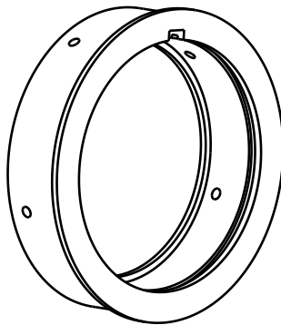
Vue isométrique 2 (de dos) Echelle : 1:2
