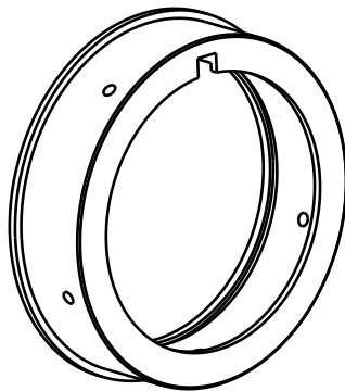
Vue isométrique (de face) Echelle : 1:2
