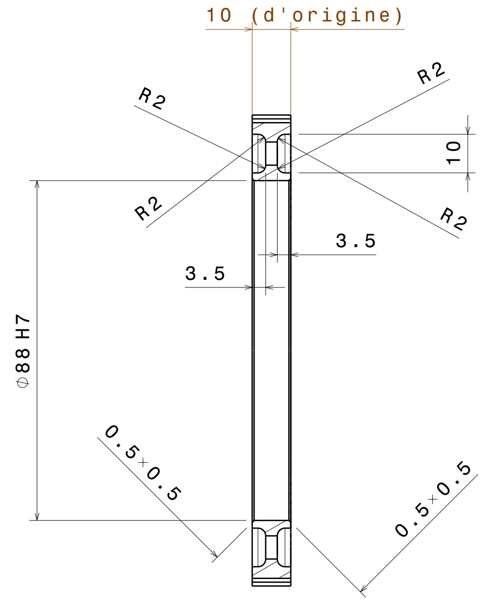
Coupe A-A Echelle : 1:1
