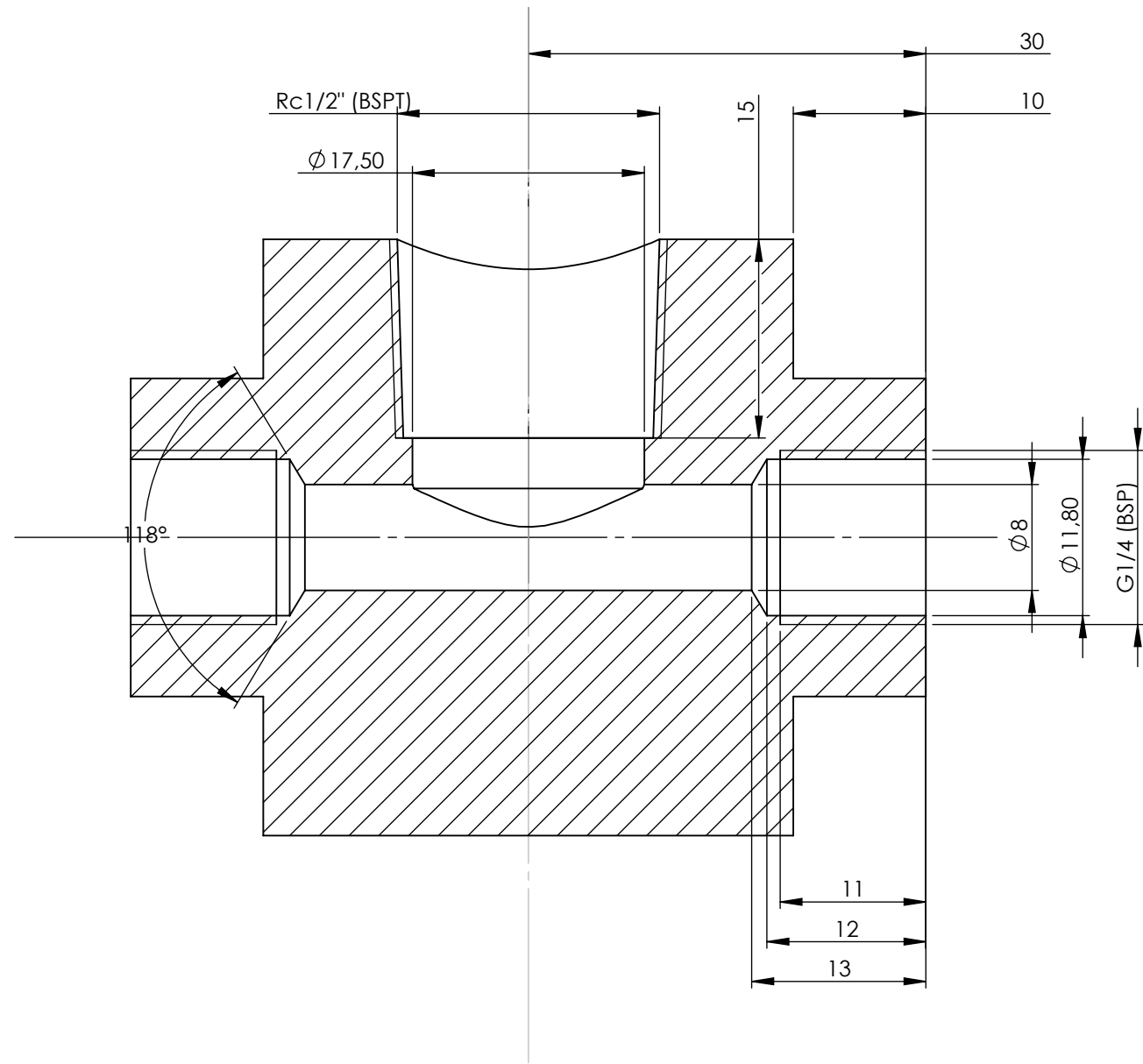
COUPE J-J
