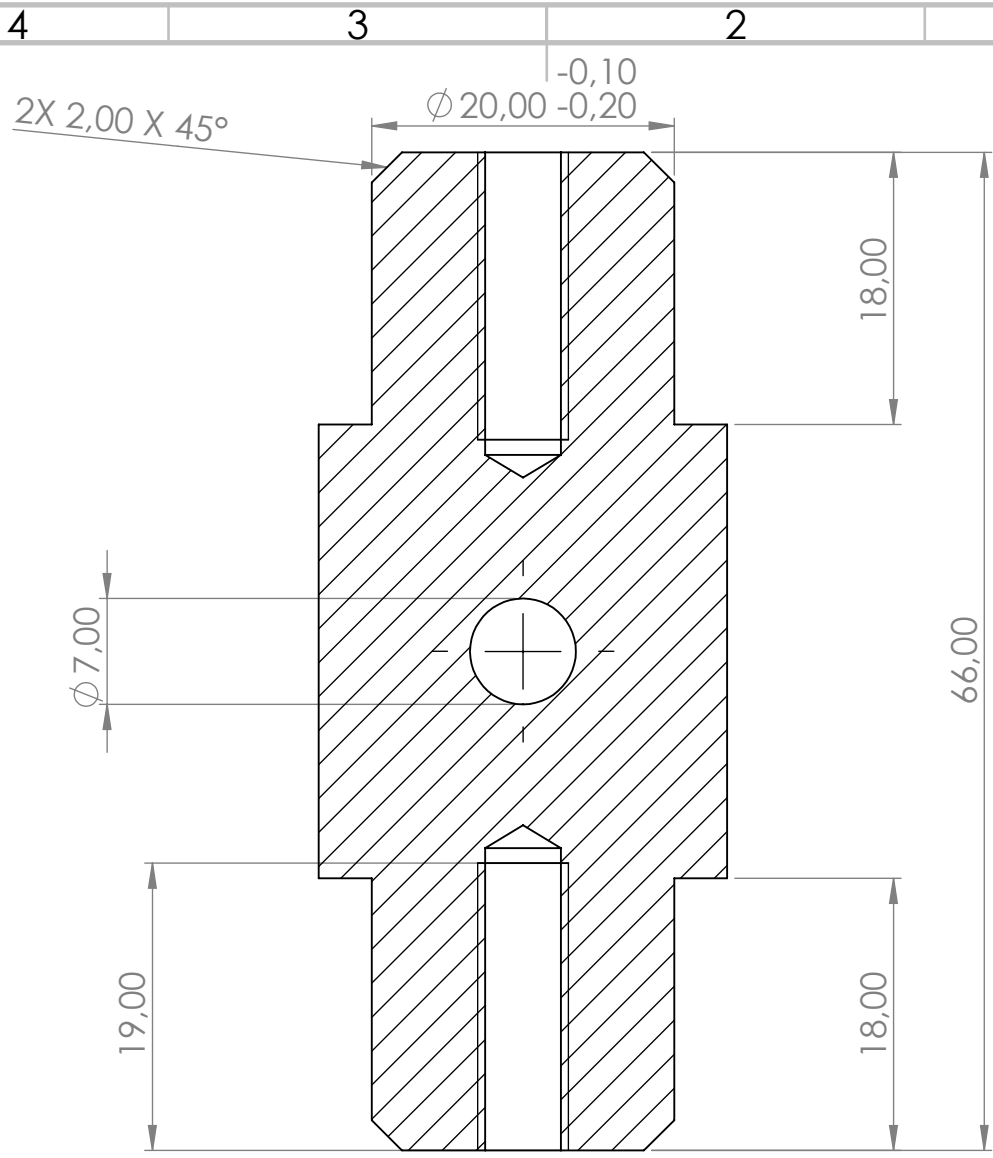
COUPE C-C
