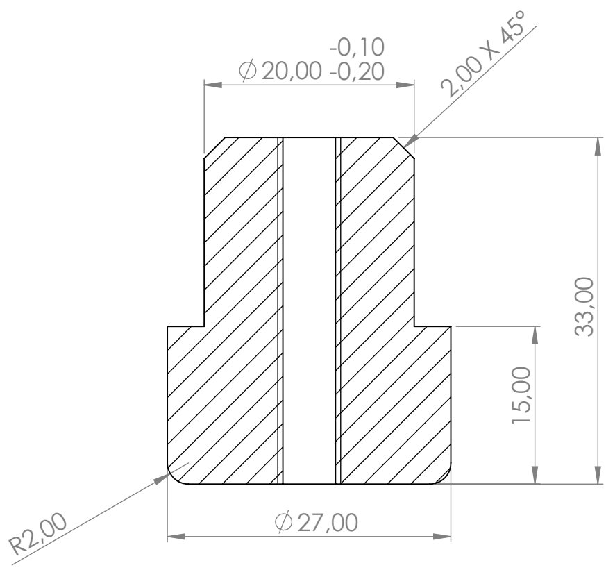
COUPE B-B
