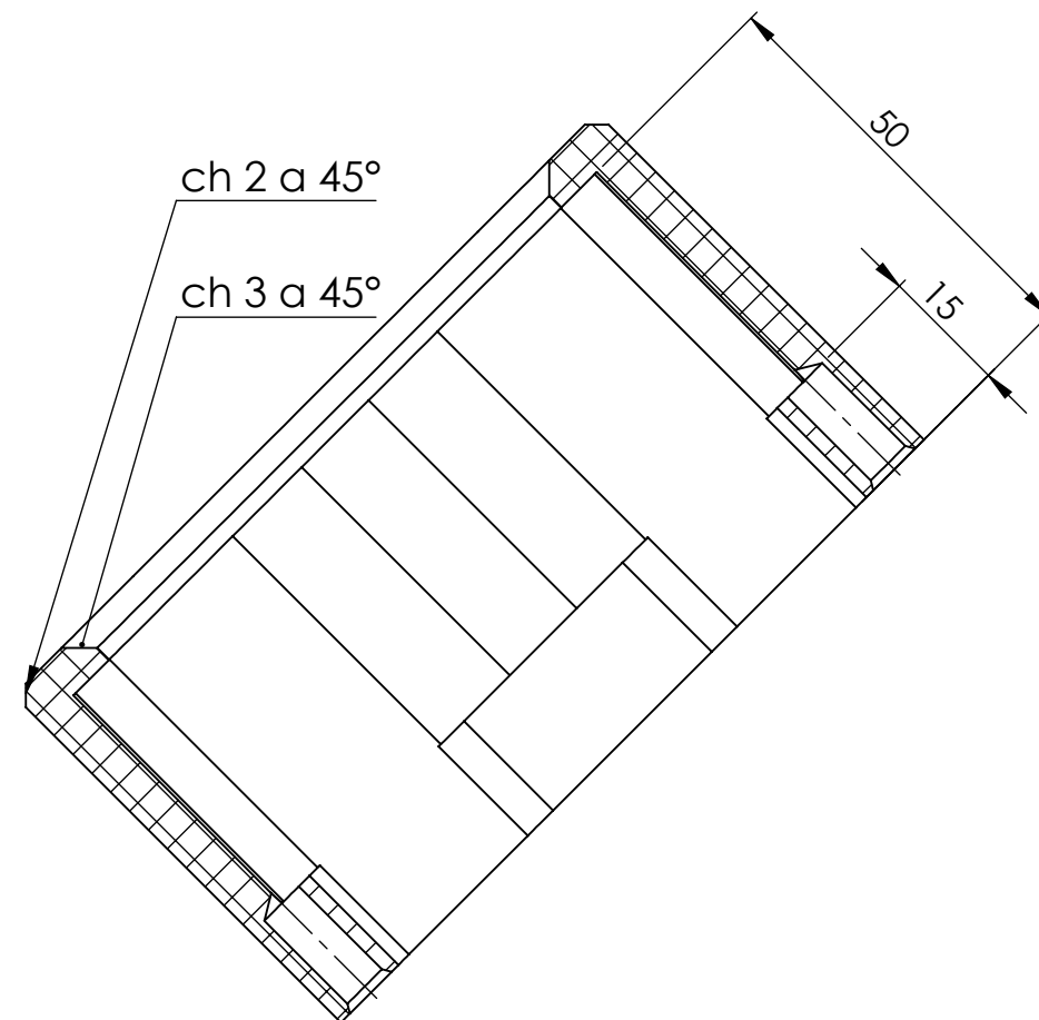
COUPE U-U ECHELLE 1 : 1
