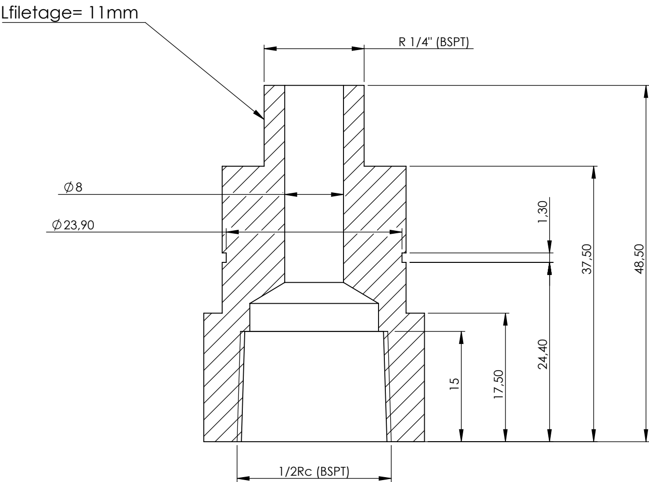
COUPE K-K
