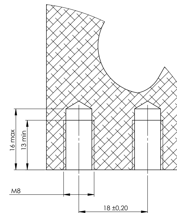
COUPE H-H
