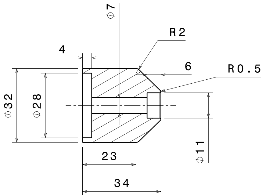
COUPE A-A
