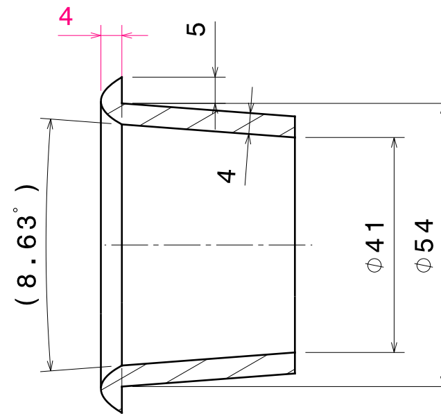
Coupe C-C Echelle : 1:1
