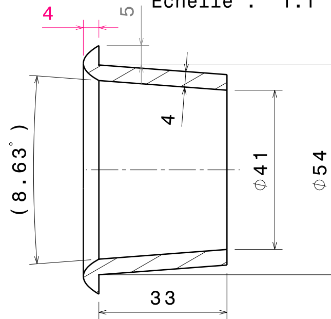
Coupe A-A Echelle : 1:1
