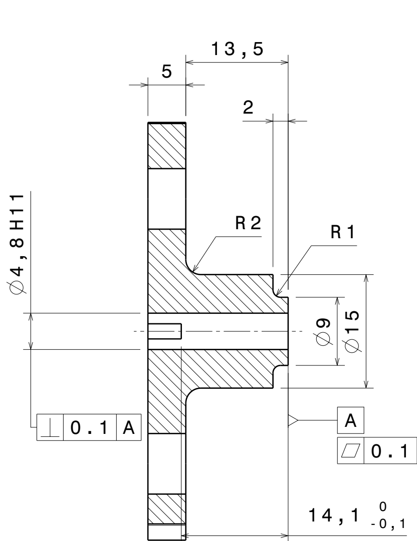
Coupe A-A
