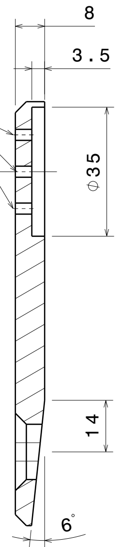
Section A-A Scale : 1:1
