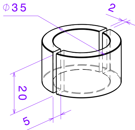
DETAIL DEUX DEMI RONDELLE
