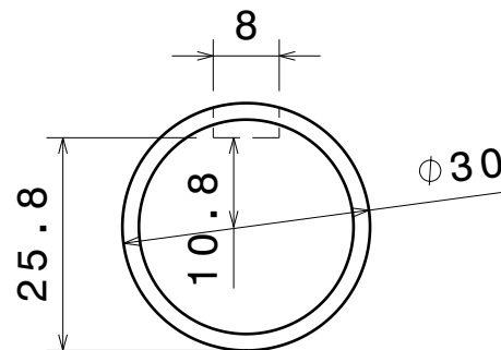
Vue de face Echelle : 1:5
