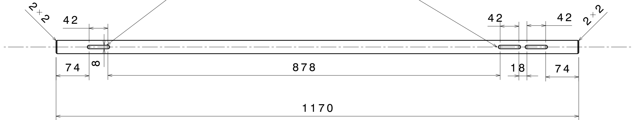
Vue de face Echelle : 1:5
