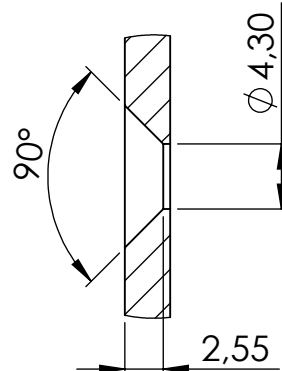
DÉTAIL C ECHELLE 2 : 1
