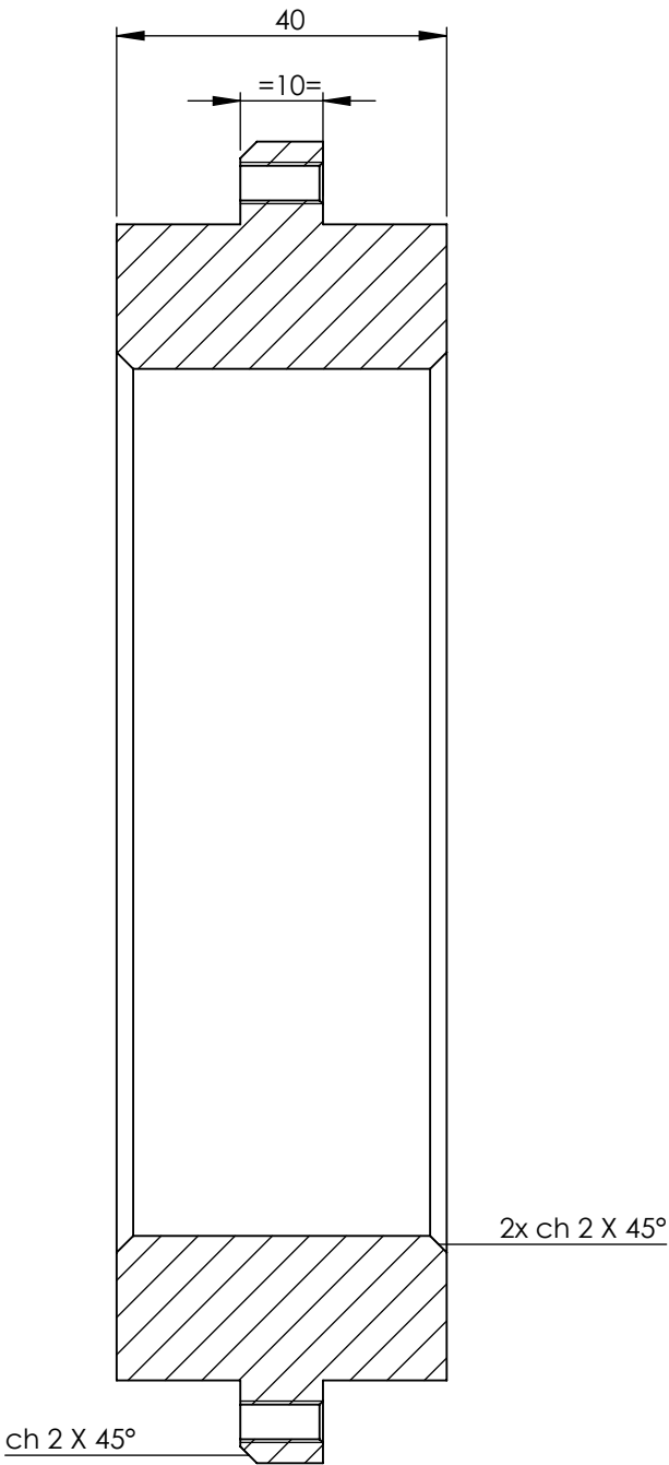
COUPE H-H ECHELLE 1 : 1
