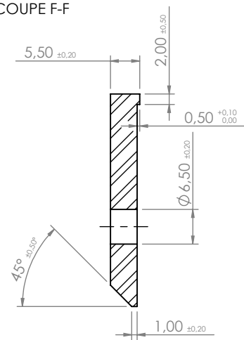
COUPE F-F
