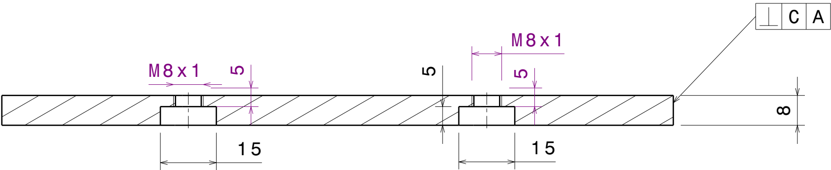
Coupe A-A Echelle : 1:1
