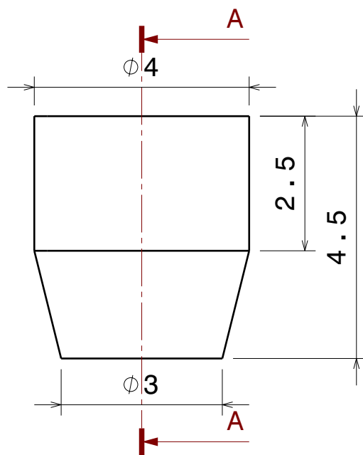
Vue de face Echelle : 10:1
