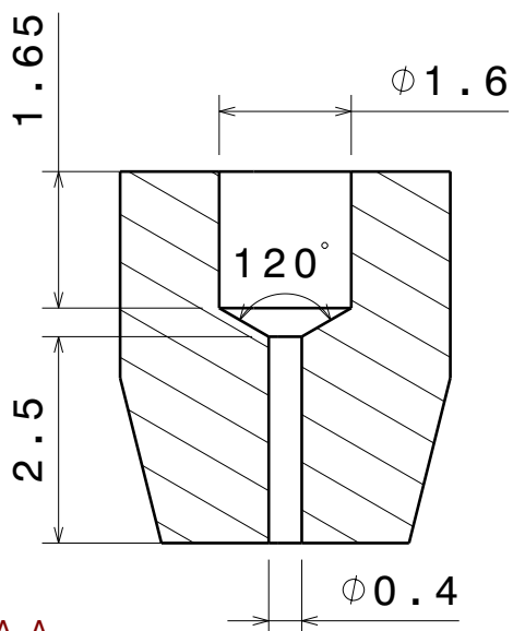
Coupe A-A Echelle : 10:1
