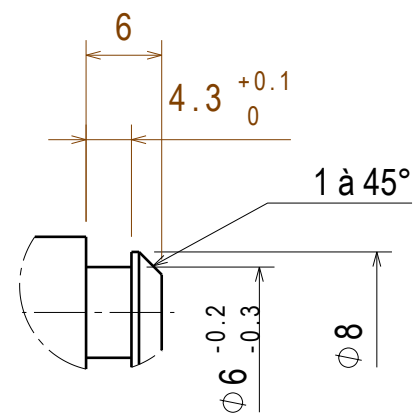
Détail A Echelle : 2:1
