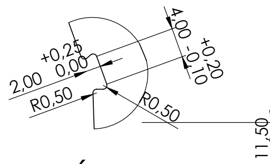
DÉTAIL A ECHELLE 2:1
