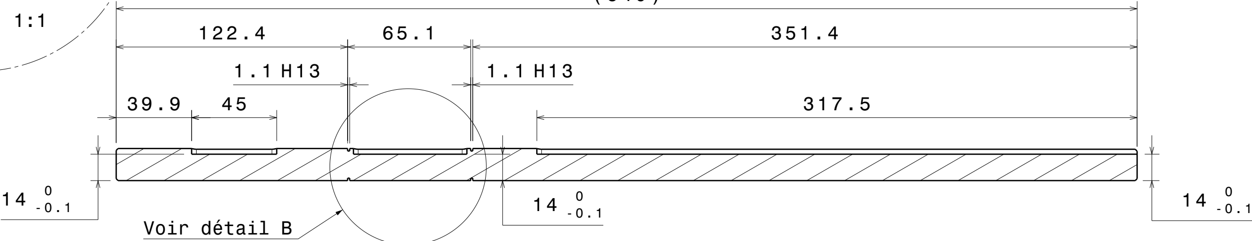
Coupe A-A Echelle : 1:2
