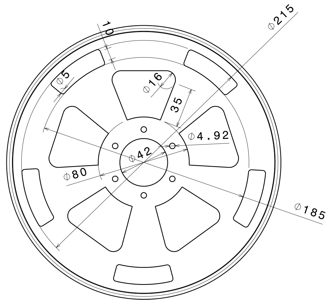
Vue de dessous Echelle : 1:2
