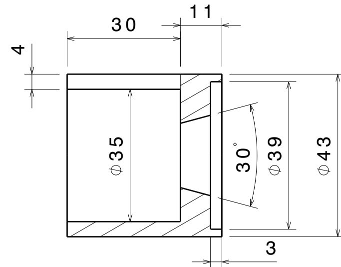
Coupe A-A Echelle : 1:1
