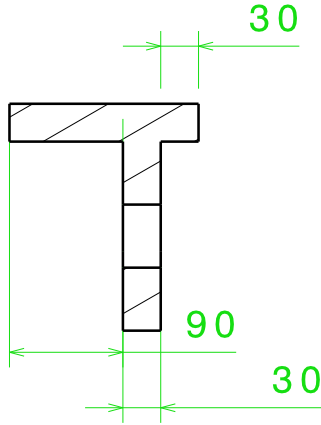
Coupe A-A
