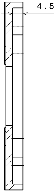
Coupe A-A
