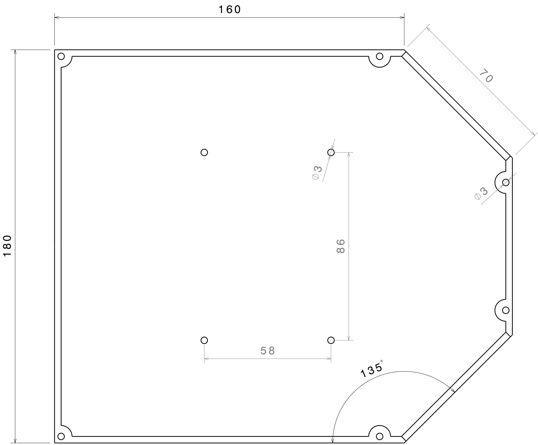
Front view Scale: 1:1
