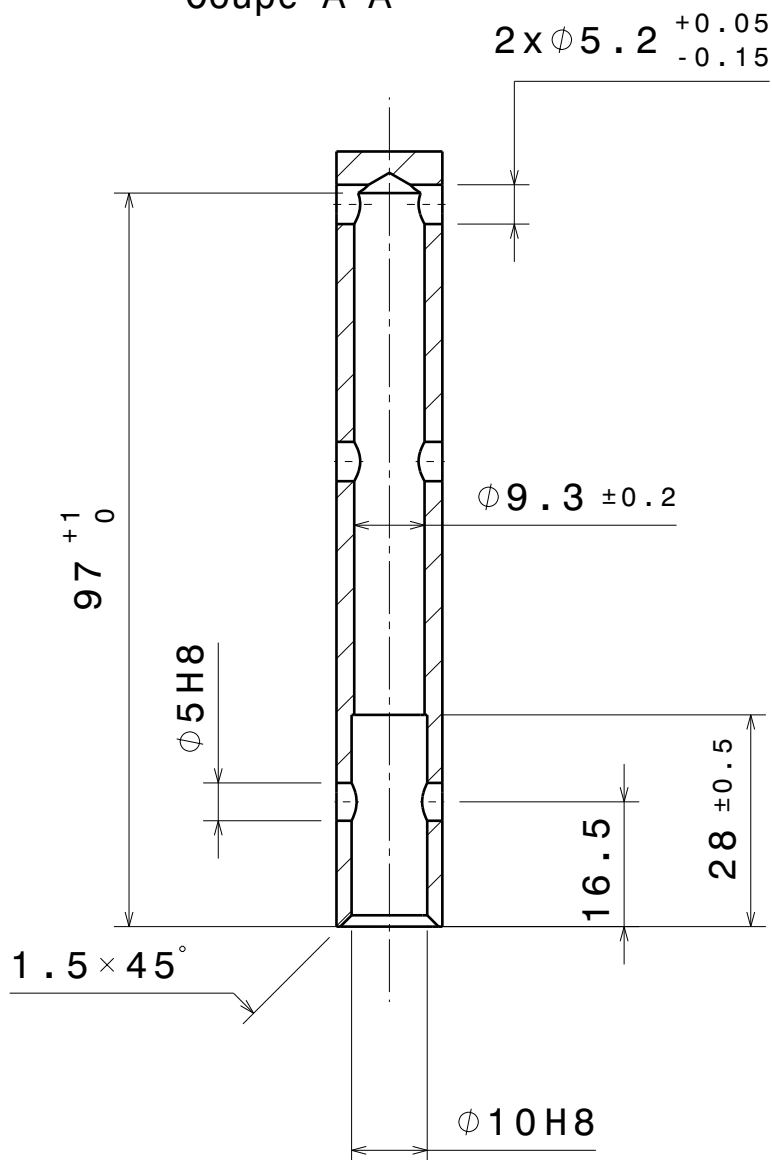
Coupe A-A
