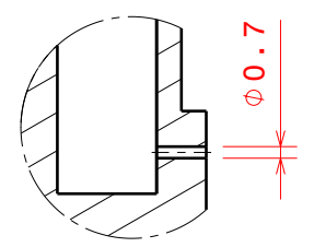
Détail C
