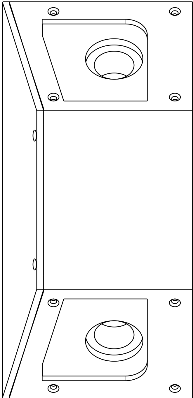
Right view Scale: 1:1
