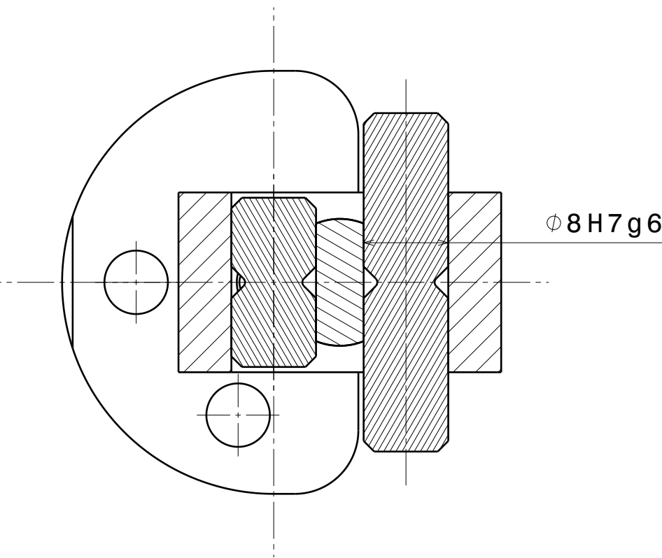
Coupe B-B
