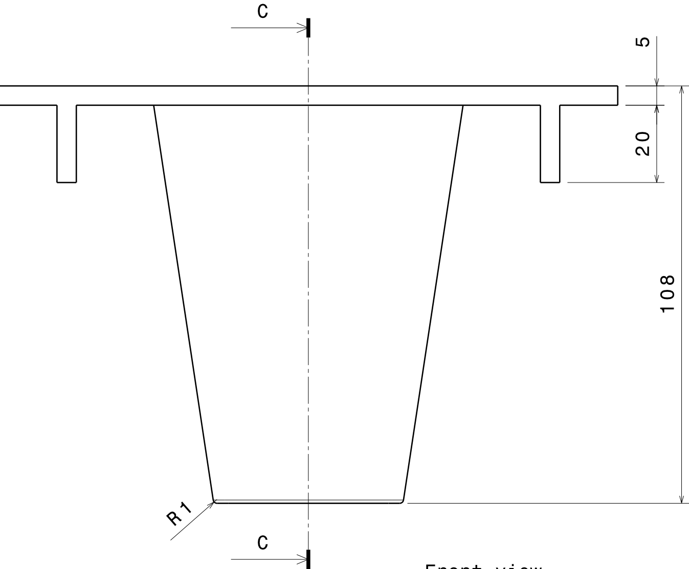
Front view Scale: 1:1
