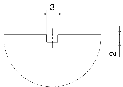
Detail G Scale: 2:1
