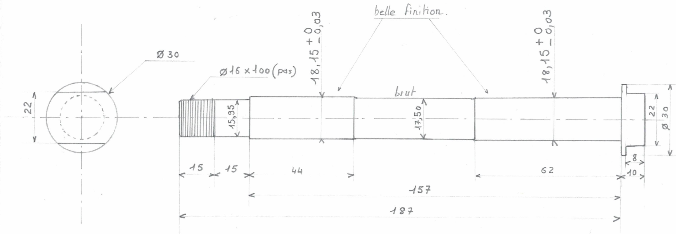
VUE DE DROITE
