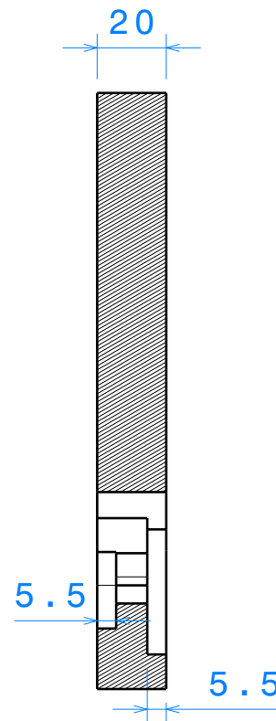
Section view A-A Scale: 1:2
