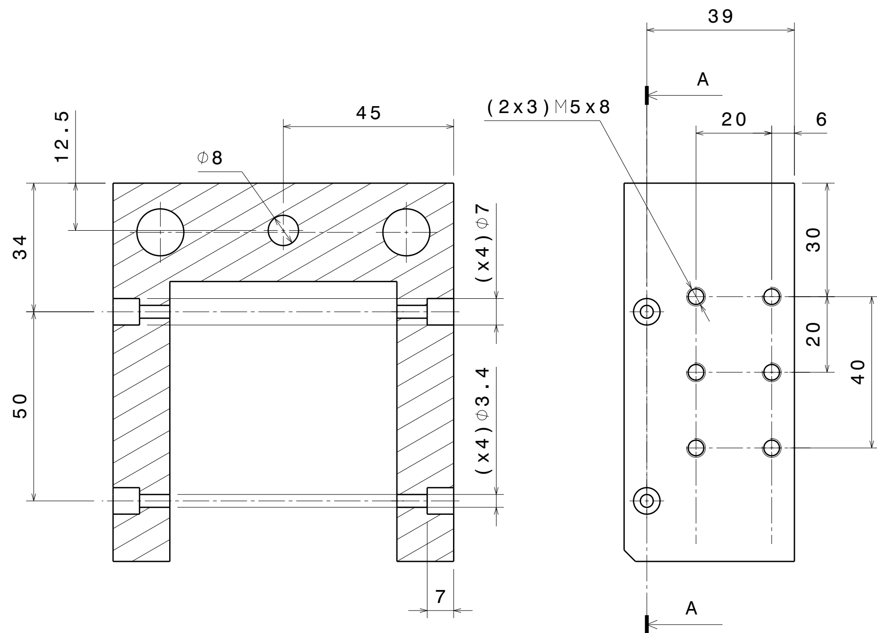
Coupe A-A
