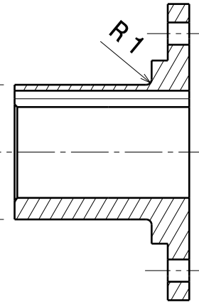
Coupe A-A Echelle : 1:1
