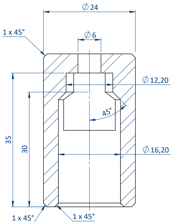
COUPE A-A
