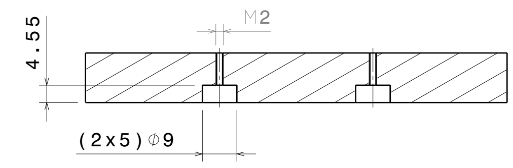
Coupe B-B Echelle : 1:1
