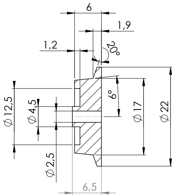
COUPE D-D
