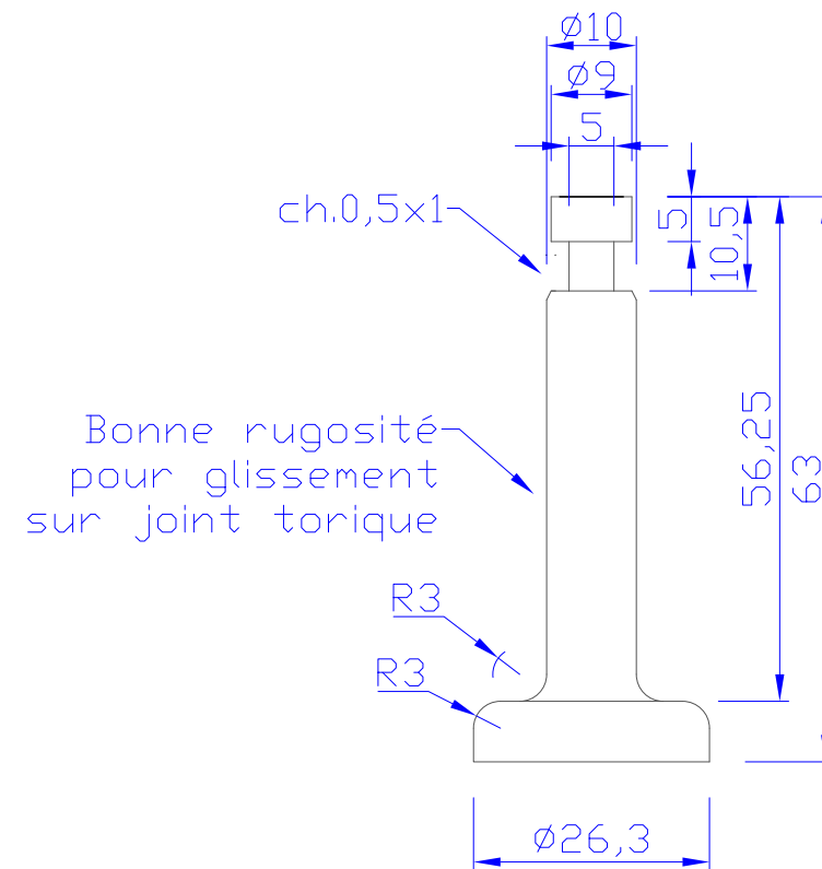
Rep2 - Obturateur Matière: INOX Quantité: 1
