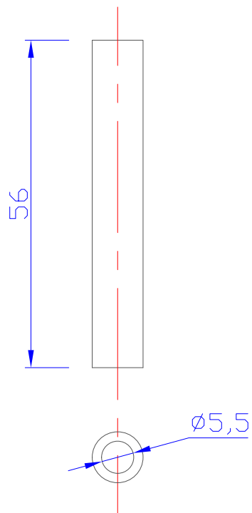
Rep3 - Support vérin Matière: INOX Quantité: 2
