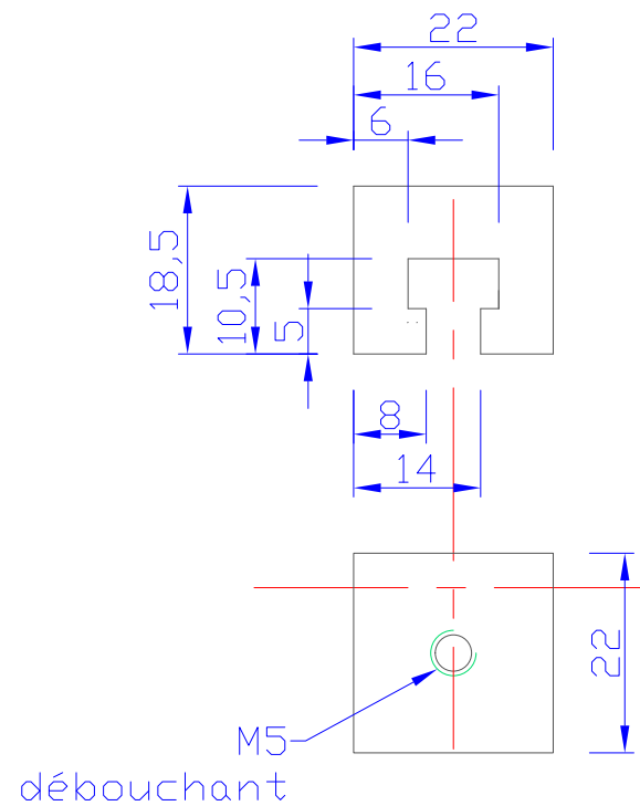
Rep1 - Accouplement Matière: INOX Quantité: 1
